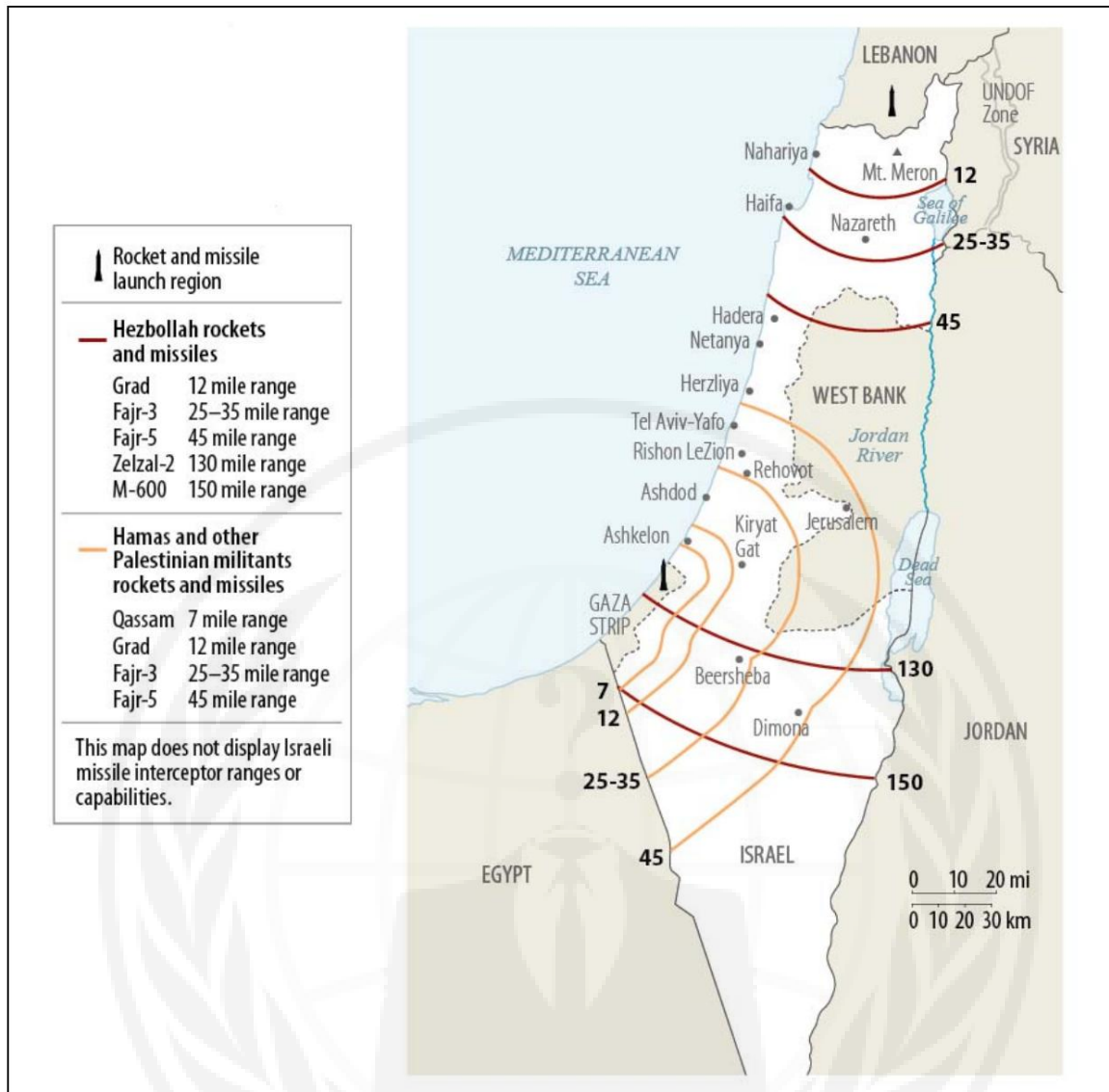
شکل 5. برد احتمالی راکت ها و موشک های گروه های متحد ایران (تا فوریه 2012)
